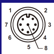
A-Coding M12
