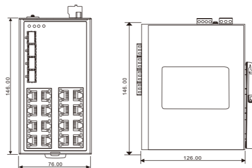
IG(P)S-3164GP-LA
