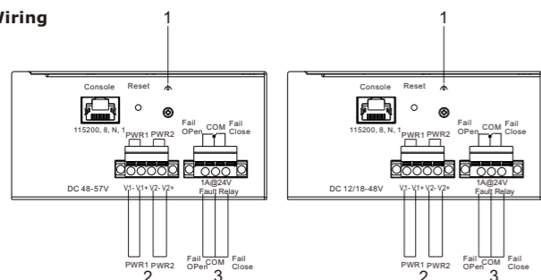
IGPS-3084GP-LA/IGPS-3164GP-LA IGS-3084GP-LA/IGS-3164GP-LA
