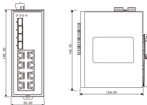
IG(P)S-3084GP-LA
